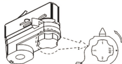
4- Drähte-Adapter
