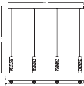
DECOR TWIRL PENDANT 4XGU10 PAR11 BG
