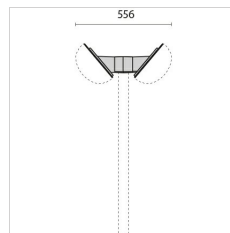
000810 Doppelter, 40° geneigter Sockel f. 42 mm Ø Mast Schwarz
