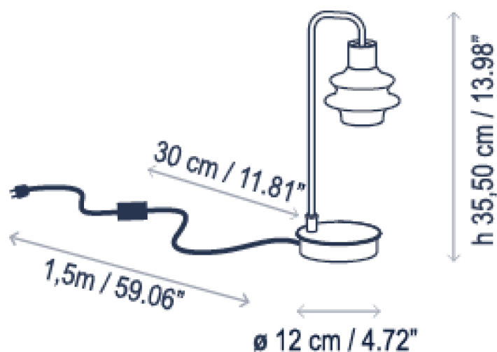
Interruptor en el cable / Through cord switch
