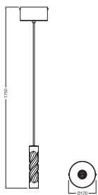
DECOR TWIRL PENDANT GU10 PAR11 BG
