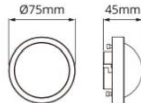
Abmessungen Lichtquelle
