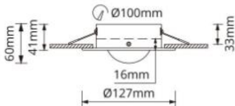
Abmessungen Leuchte
