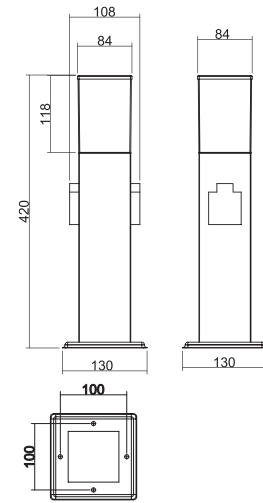
Μαßeinheit/Unit of measure/ Unité de mesure: mm
