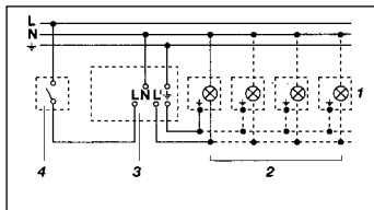
2. Lampă cu conductorul neutru disponibil
