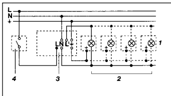
1. Lampă fără conductorul neutru disponibil
