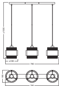
DECOR HORNET PENDANT LINEAR 3XE27
