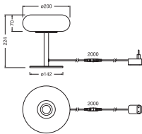
DECOR LUNEA TABLE 8W CCT DIM WT
