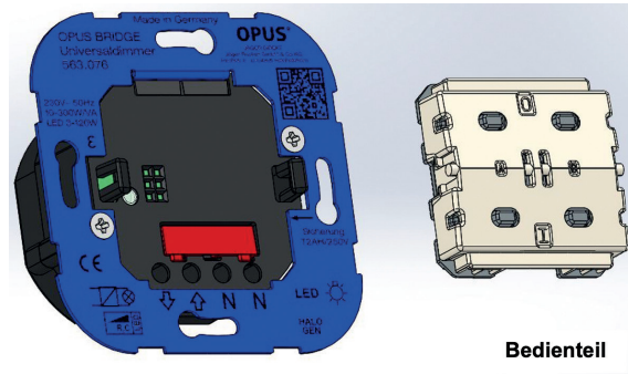
Leistungsteil
