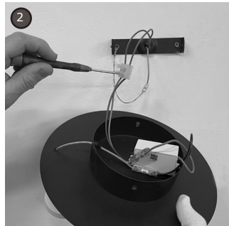
Led COB 16W - 350mA -2100 Lm emessi - 3000°K - CRI>85 I Classe IP 20 - Fatto in Italia
