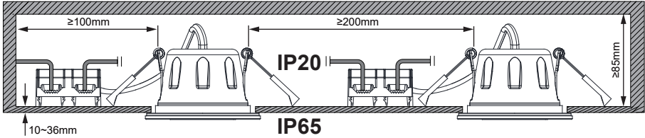
MM76753,MM76754,MM76755,MM76756 ohne Abstandshalter LA8125
