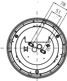
Ø300
