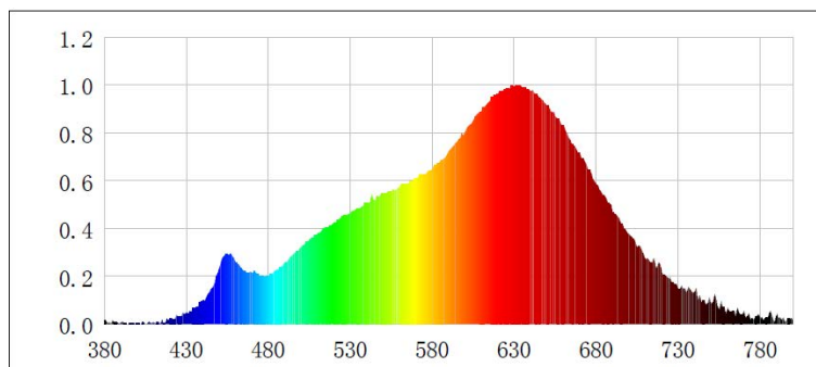
Lichtspektrum / Light spectrum Bei CCT 2700K / at CCT 2700K
