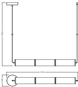
DECOR SQUEEZE PENDANT 30W 840
