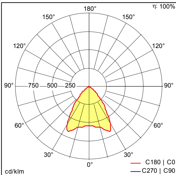
D35587AA_MIRL_MINI_EP_LED1200-830_LDO.ltd (vorläufige Messung)
