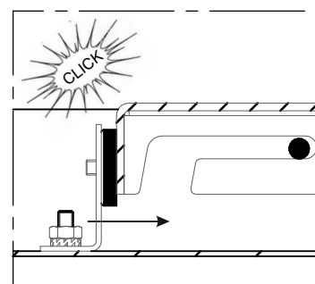
DETTAGLIO C
