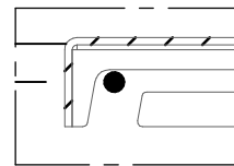
DETTAGLIO B
