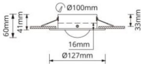
Abmessungen Leuchte
