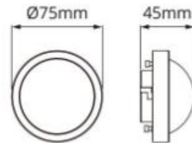
Abmessungen Lichtquelle
