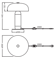
DECOR ARC TABLE 4XE14 DIM
